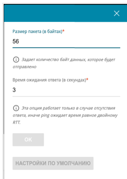
Рисунок 140. Страница Система / Пинг . Окно дополнительных настроек.
