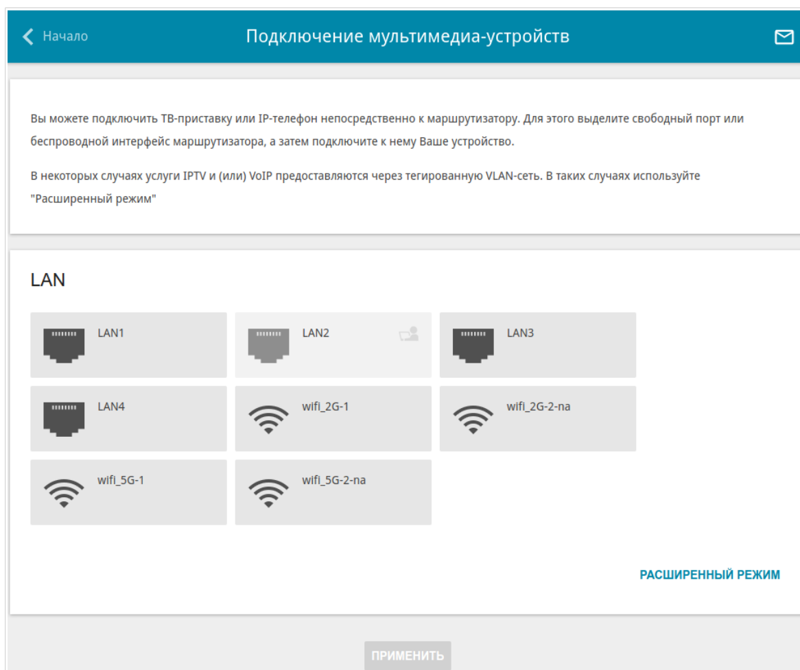
Рисунок 42. Мастер подключения мультимедиа-устройств. Простой режим.
