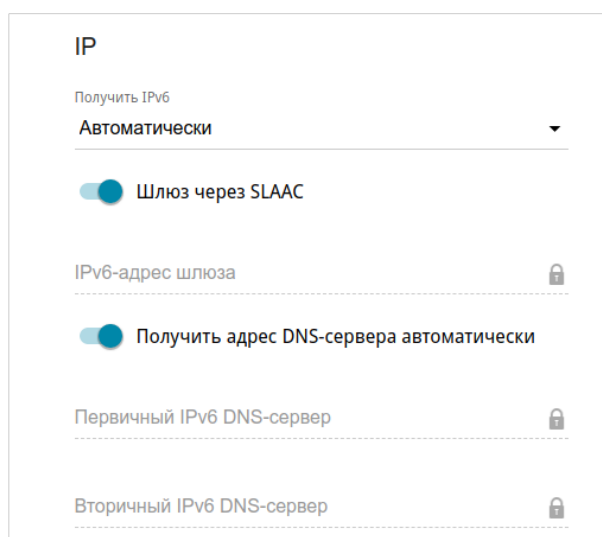
Рисунок 72. Страница добавления соединения типа PPPoE IPv6. Раздел IP.
