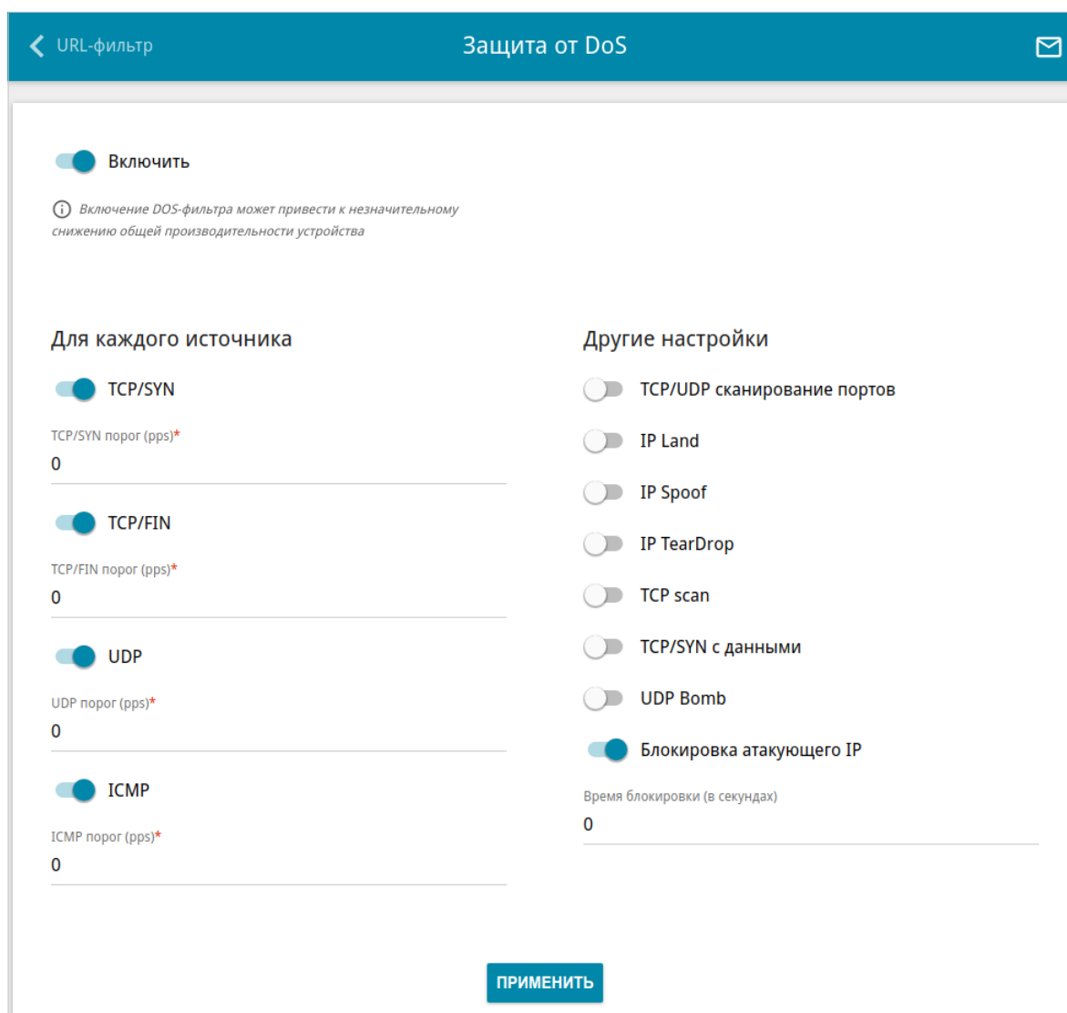
Рисунок 134. Страница Межсетевой экран / Защита от DoS .
