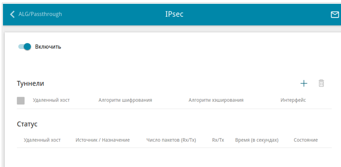
Рисунок 122. Страница Дополнительно / IPsec .
