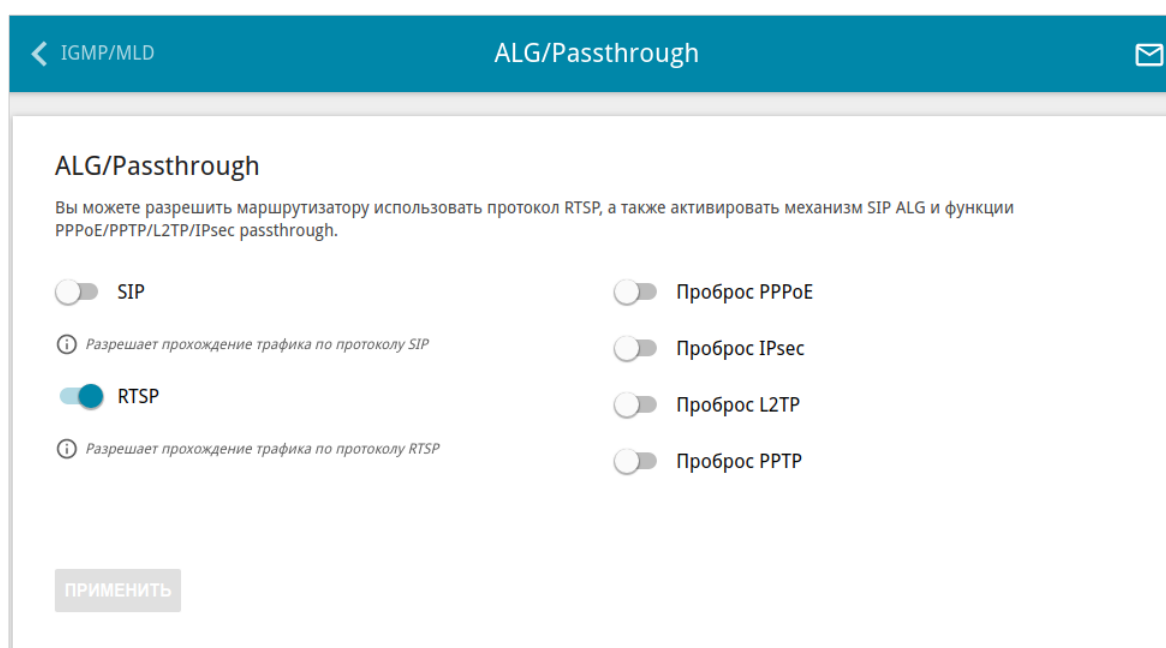
Рисунок 121. Страница Дополнительно / ALG/Passthrough .
