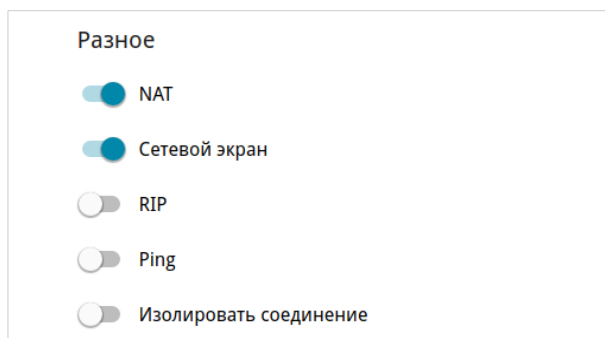
Рисунок 57. Страница добавления соединения типа Статический IPv4 . Раздел Разное .
