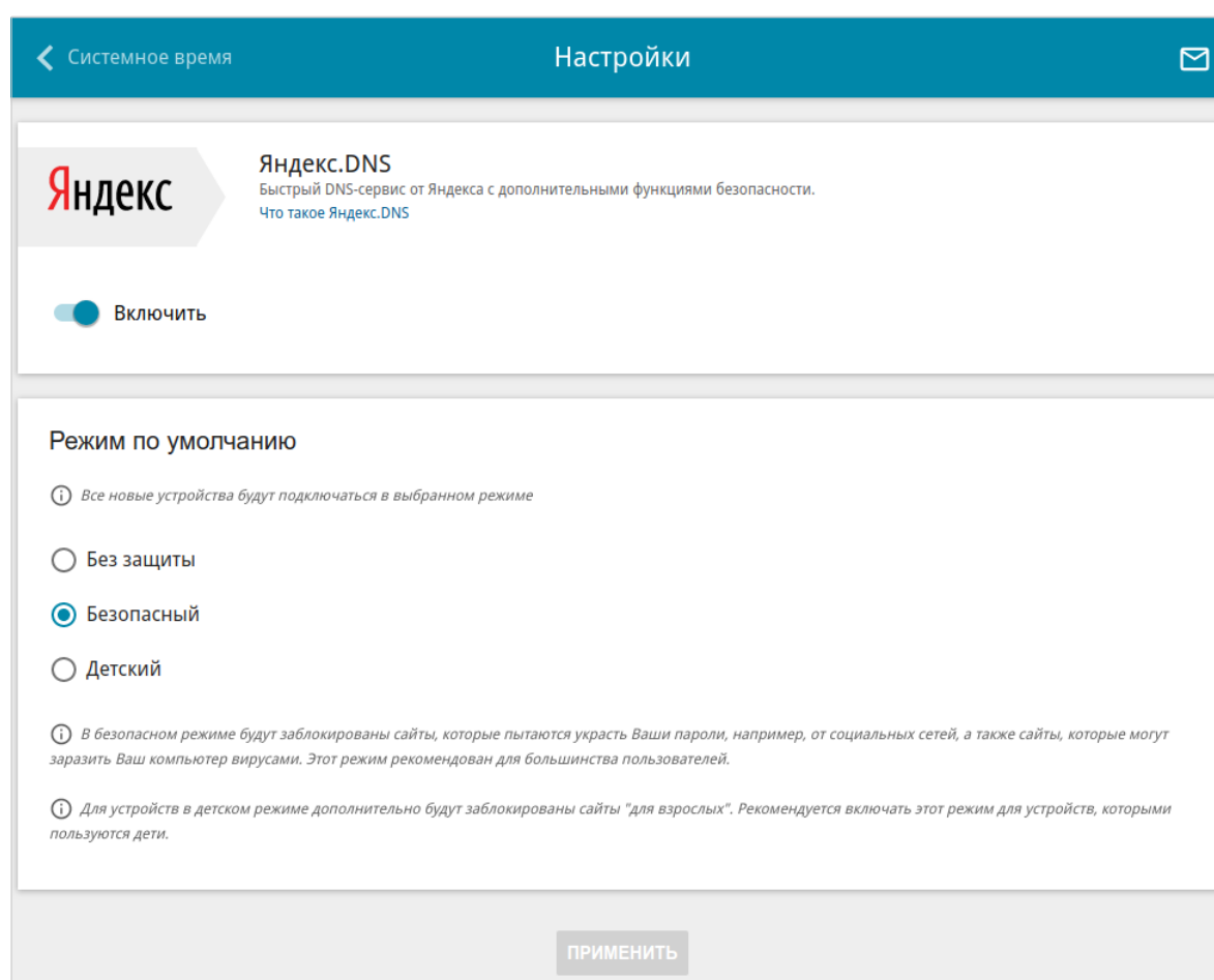
Рисунок 145. Страница Яндекс.DNS / Настройки .
