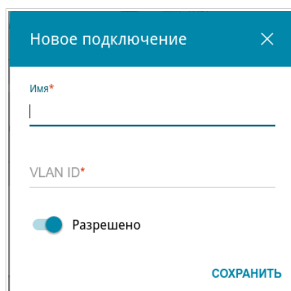
Рисунок 44. Добавление подключения.
