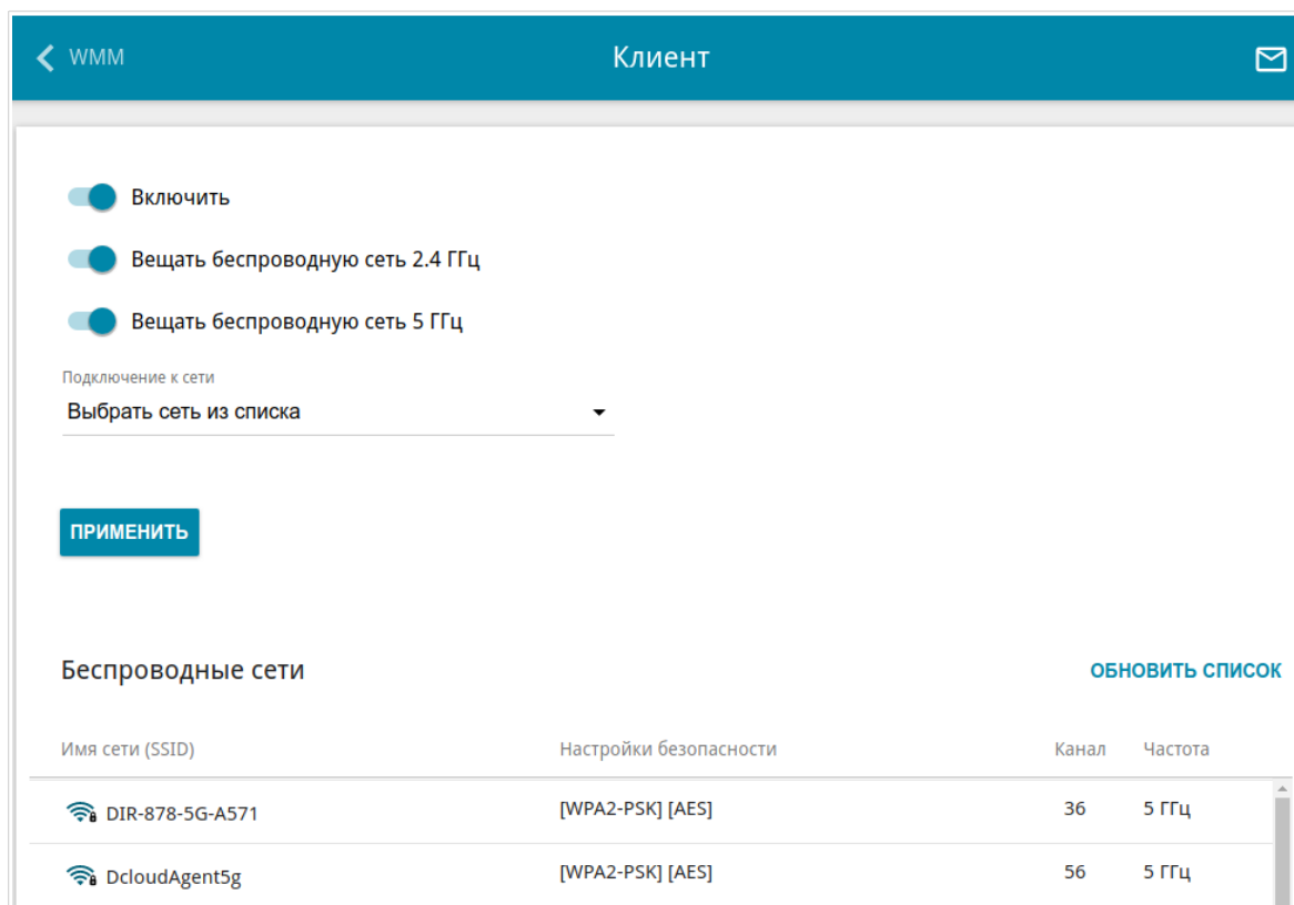
Рисунок 93. Страница для настройки маршрутизатора в качестве клиента.
