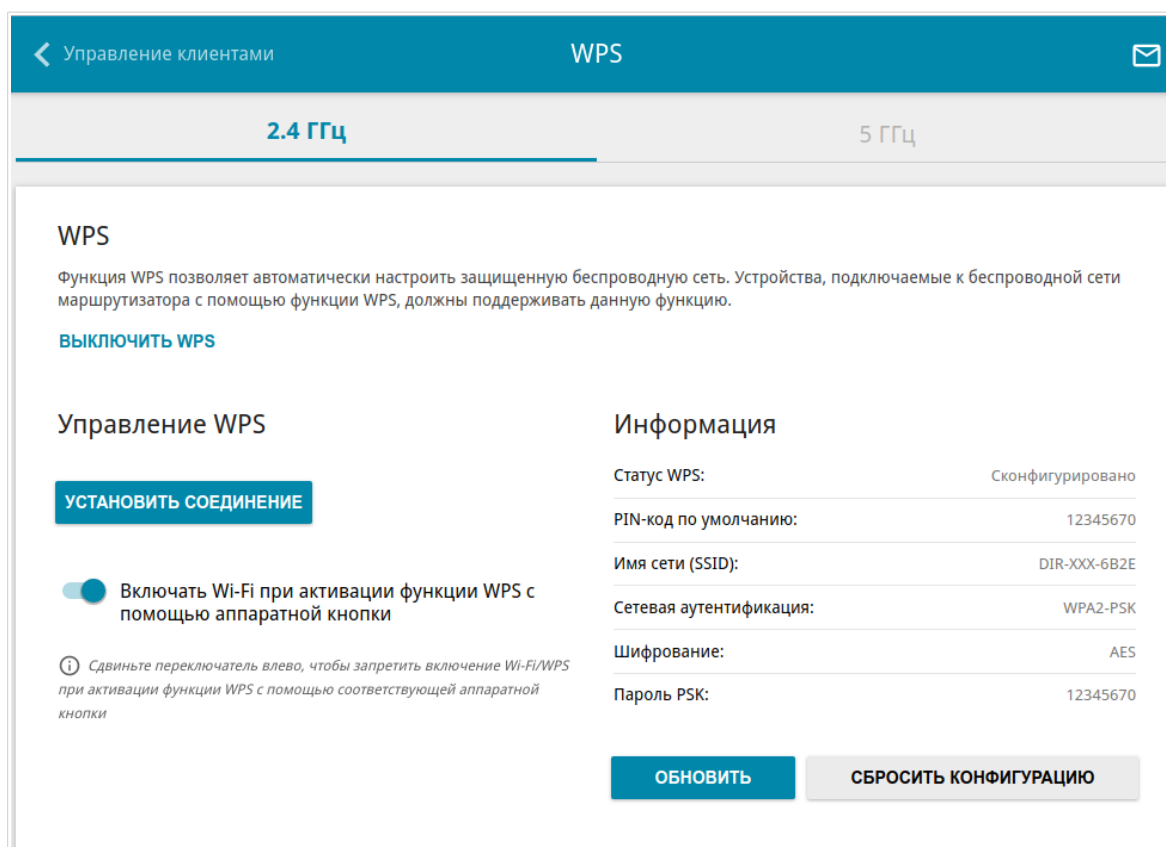
Рисунок 90. Страница для настройки функции WPS.
