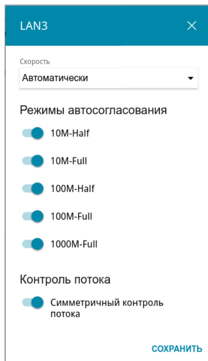
Рисунок 107. Окно изменения настроек порта маршрутизатора.
